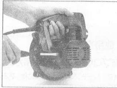
カーボンブラシの取り替え 図6
